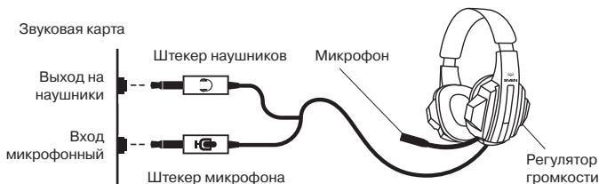
Рис. 1. Схема подключения
